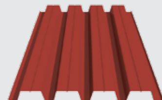
Профилированный лист МП-35x1035-B Толщина материала 0.45 - 0.9 мм
