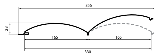
Стальной сайдинг Woodstock®-28x330 вид профилирования: гладкий
