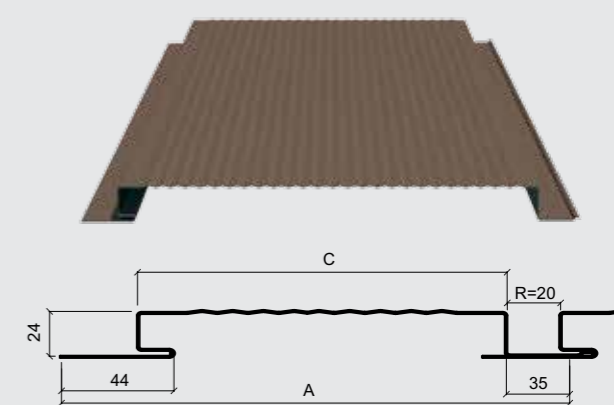
Г - вид профилирования (гладкий) В - вид профилирования (волна)
