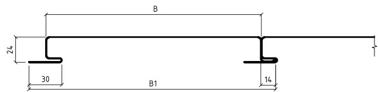
Линейные панели без руста МП ЛП-О-24xВ/0 (с открытыми торцами)
