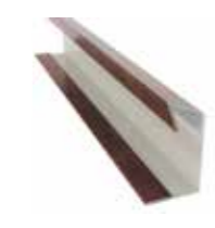
Планка начальная 22x15x3000
