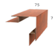
Планка угла наружного сложного 75x75x3000
