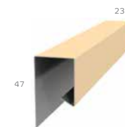
Планка завершающая сложная 30x25x3000
