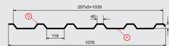
Профилированный лист МП-35x1035-А Толщина материала 0.45 - 0.9 мм
