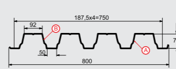
Профилированный лист Н-75x750-A,B Толщина материала 0.65 - 1.0 мм
