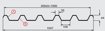
Профилированный лист С-44x1000-A Толщина материала 0.45 - 0.8 мм
