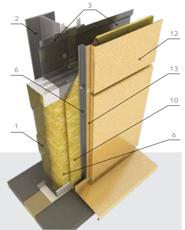
Облицовка фасадными кассетами PUZZLETON® (на примере варианта Центр)
