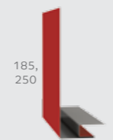
Планка карнизного свеса сложная 185x50x2000, 250x50x2000
