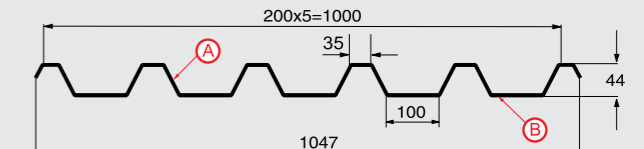
Профилированный лист С-44x1000-А Толщина материала 0.45 - 0.8 мм
