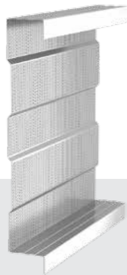
Сэндвич-профиль акустический МП СПА-100x595, МП СПА-150x595
