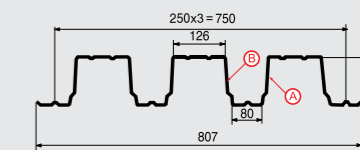
Профилированный лист Н-114x750-A,B Толщина материала 0.7 - 1.0 мм
