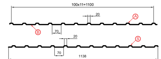
Профилированный лист С-10х1100-А,В,С Толщина материала 0.4 - 0.7 мм Производится в СФО
