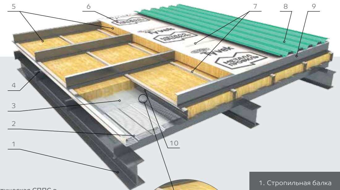
Акустическая СППС в кровельной конструкции (на примере варианта с дополнительным утеплением)
